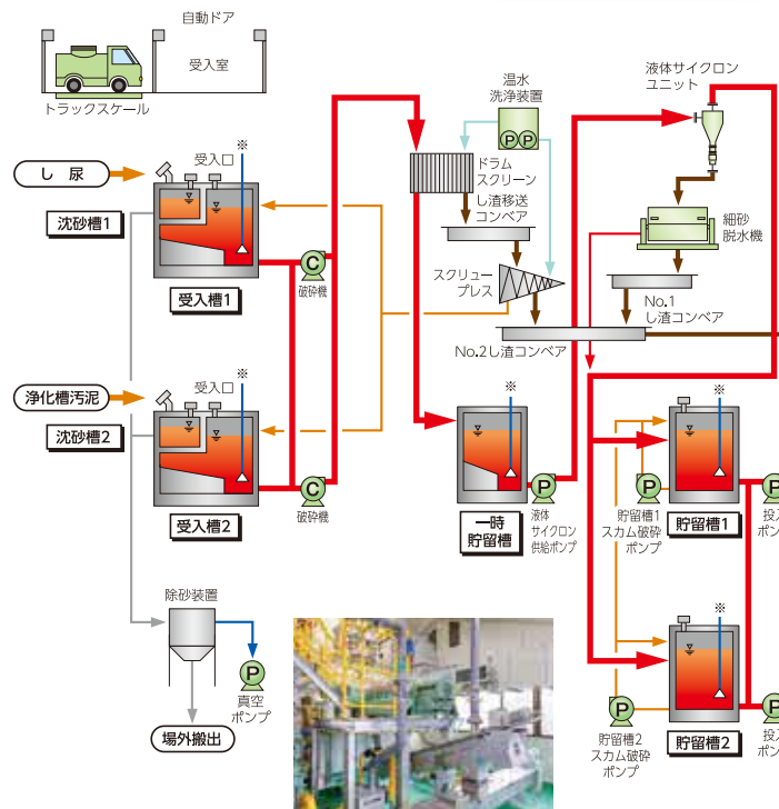
細砂除去装置
