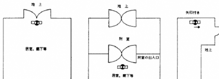
図16-8 避難口誘導灯の設置例
