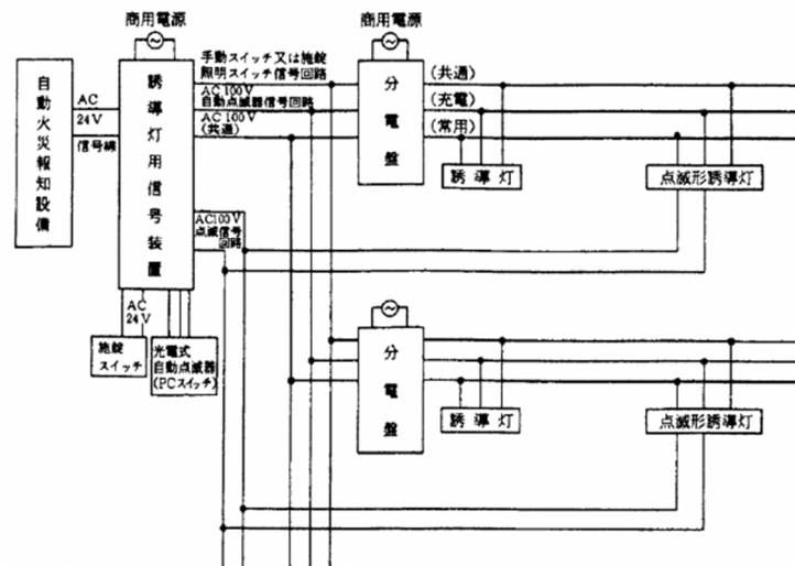
図16-23 機器結線図
