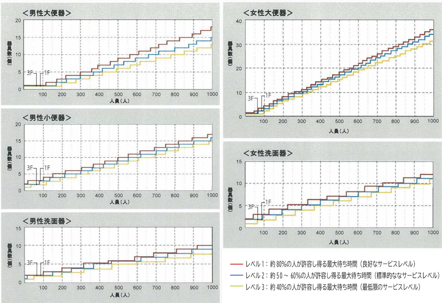
ホール算定グラフ
