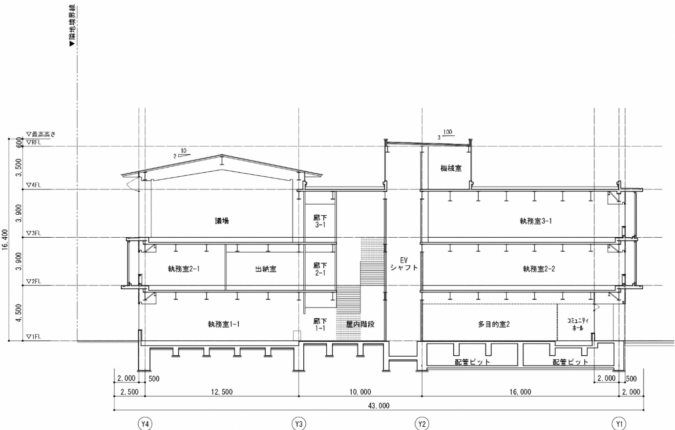
A-A' 断面図
