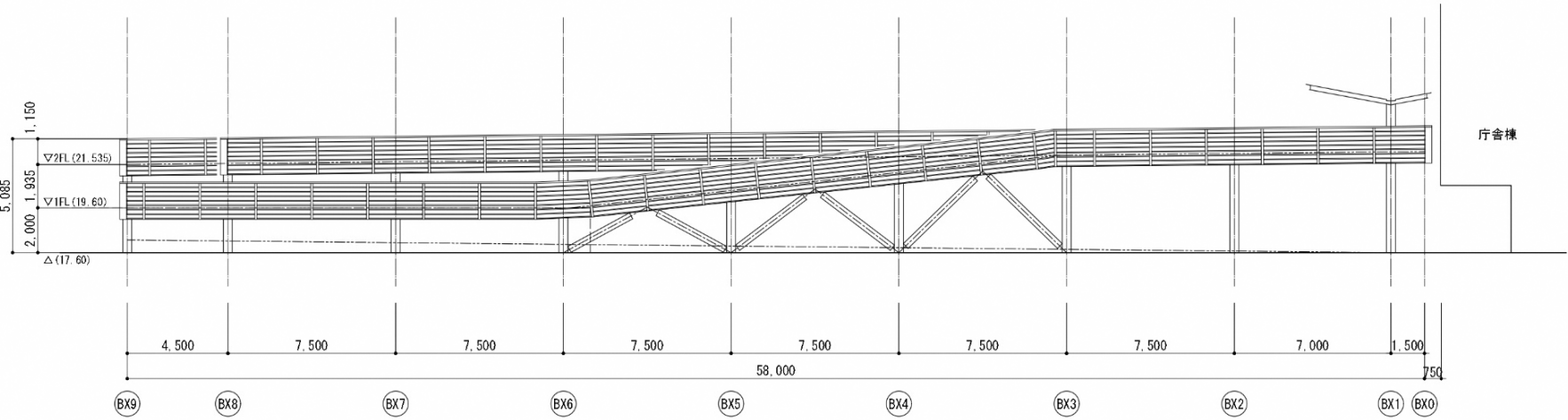
北側立面図-2
