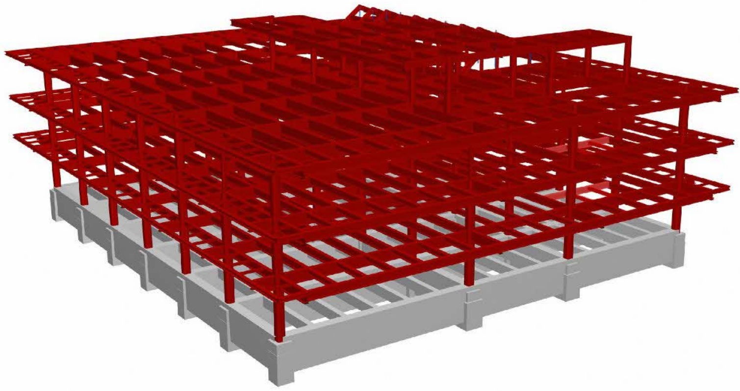
【架構パース】
