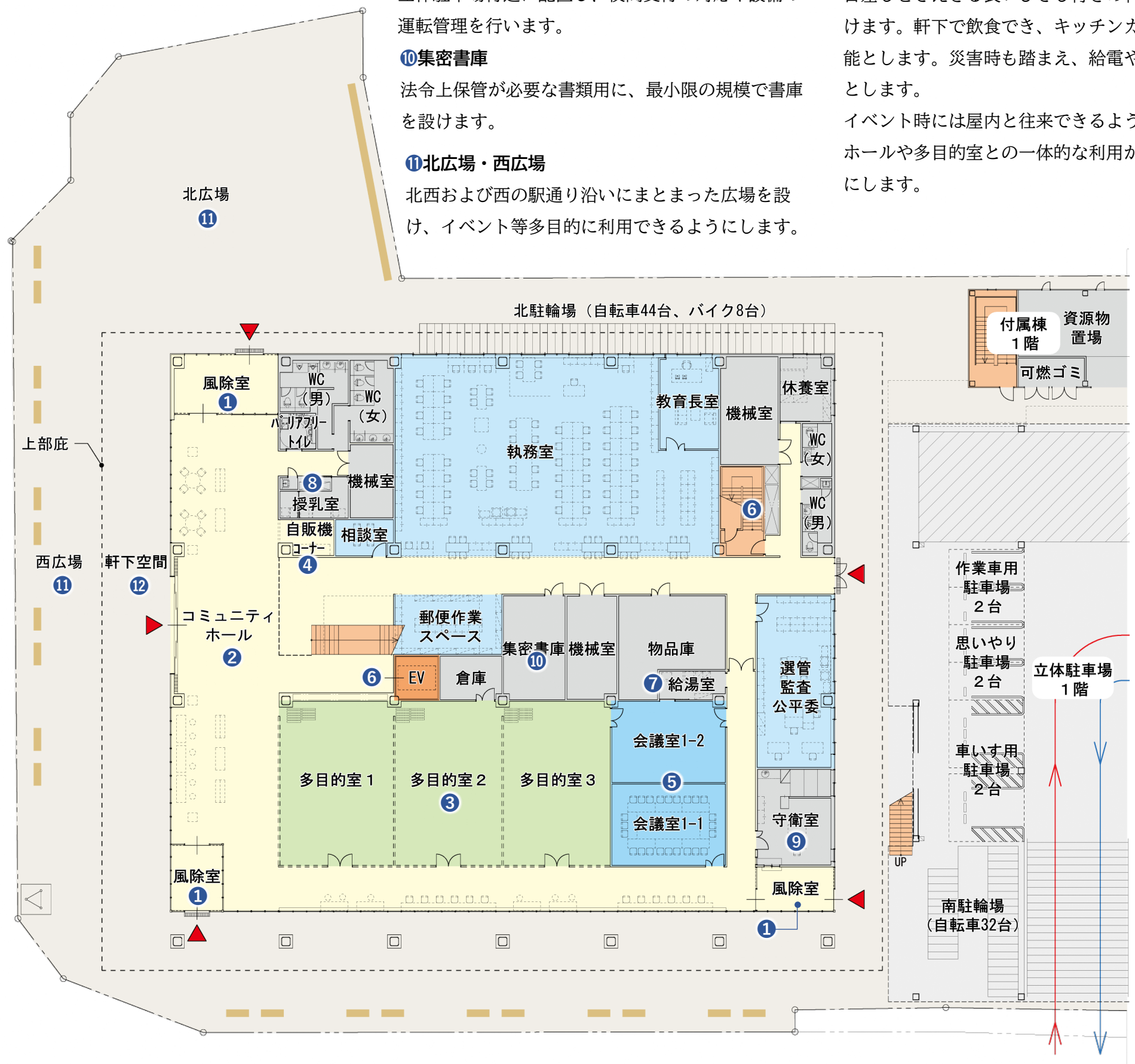
1階平面図
