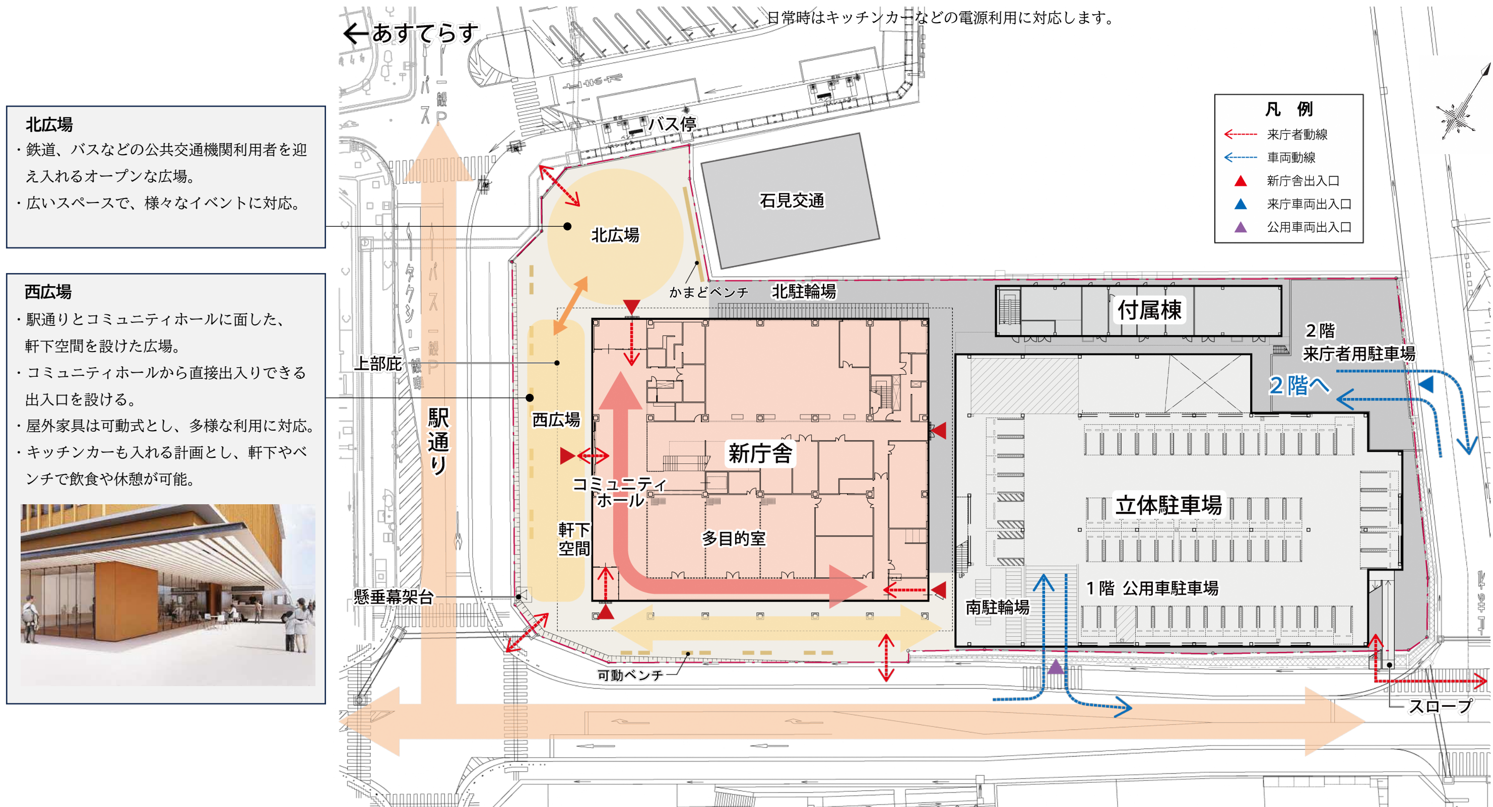
外構計画図
