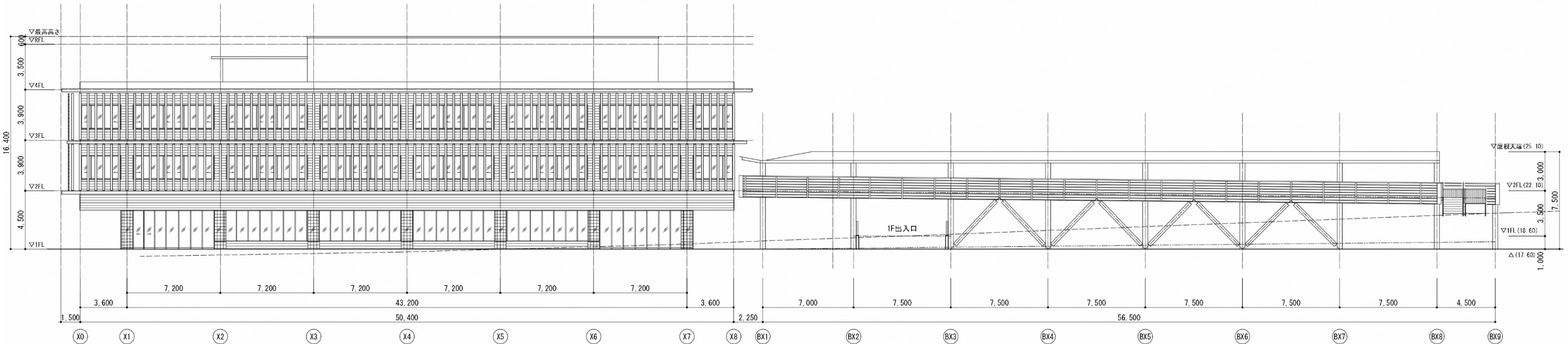
南側立面図
