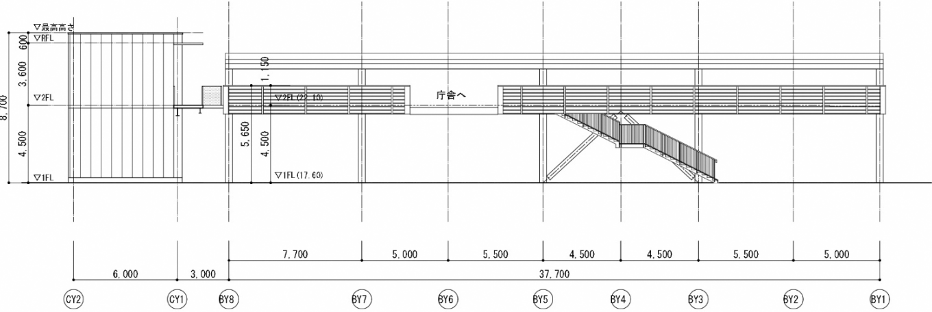
西側立面図-2
