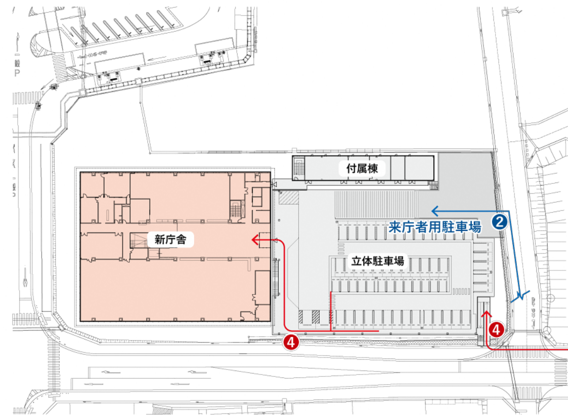
2 階平面図
