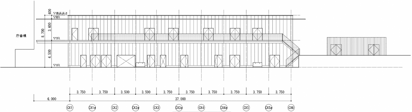
南側立面図-2
