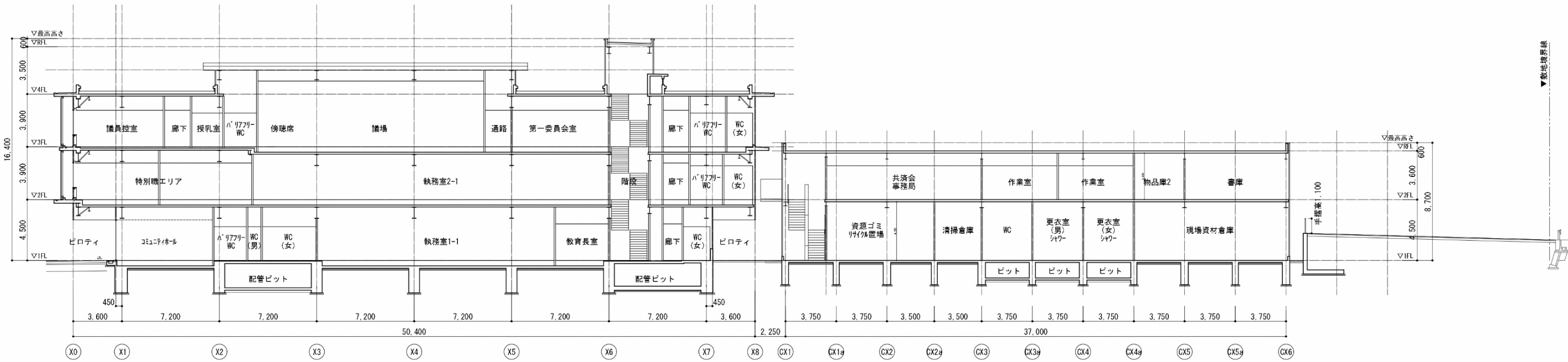
C-C' 断面図
