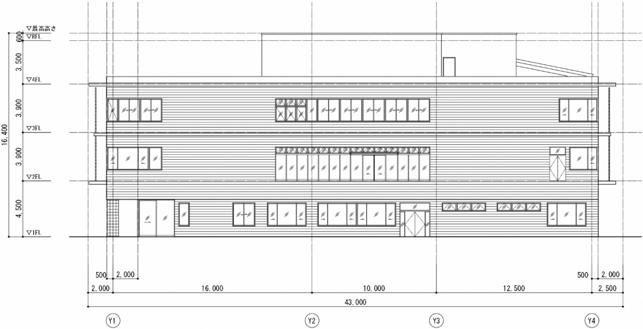
東側立面図
