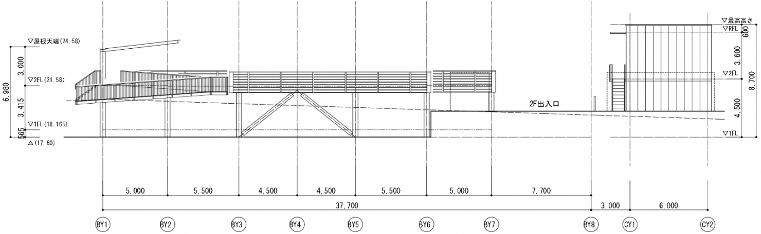
東側立面図-2
